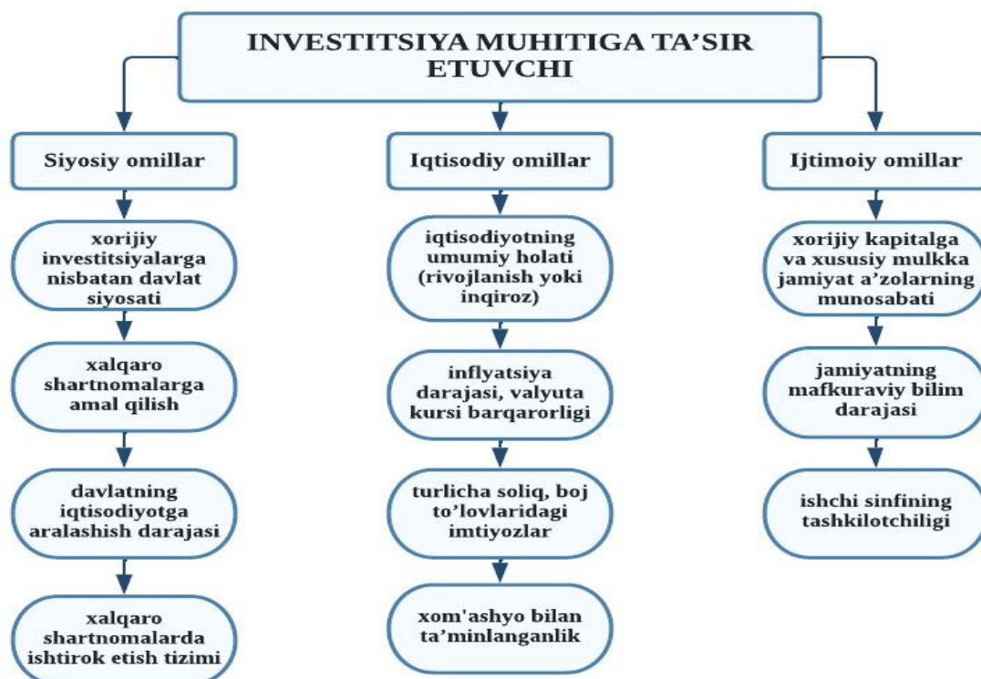
1-rasm. Mamlakat investitsiya muhitiga ta'sir etuvchi omillar [10]
